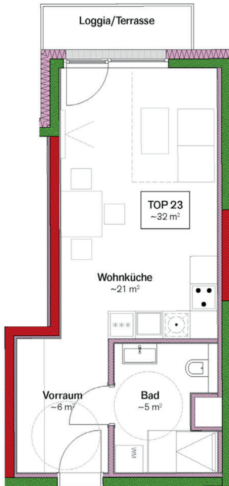
Grundriss 1. + 2. OG
